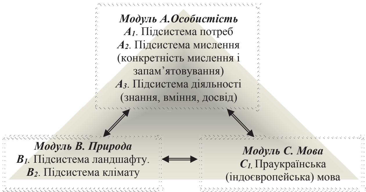
Мал. 1. Теоретична модель систем розселення і діяльності протоукраїнського населення стародавньої України та позначення цих соціальних процесів індоєвропейською мовою
